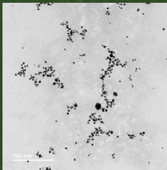
TEM Image of ALV-AU-00189
